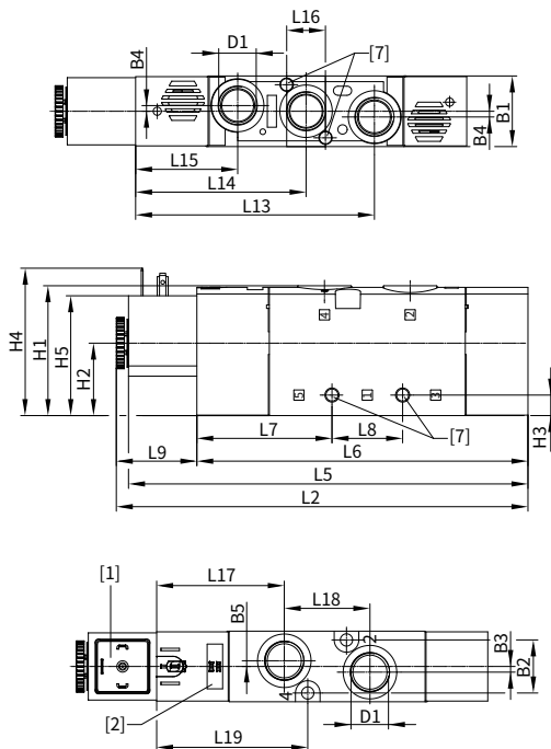
外形尺寸 - 两位五通单电控阀
